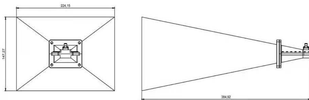
图1 天线结构尺寸图
