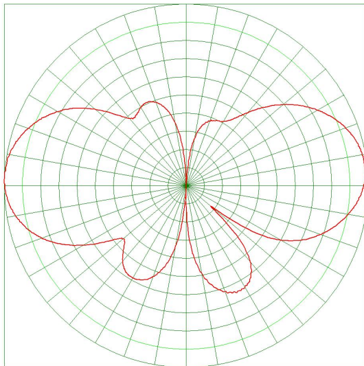
E面方向图
