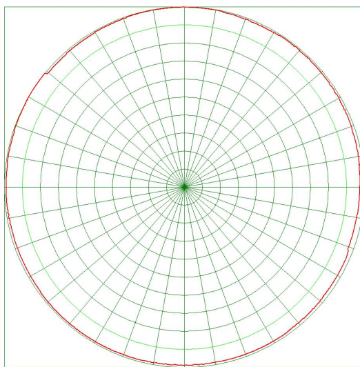
H面方向图
